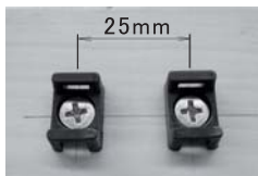
1. 25mm間隔に台座をビスで固定する
